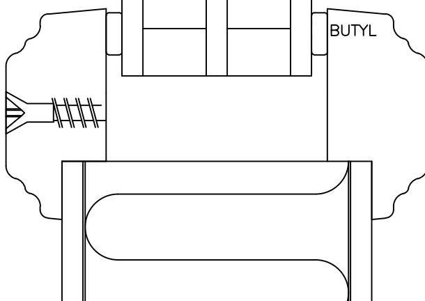
SNITT A-A
