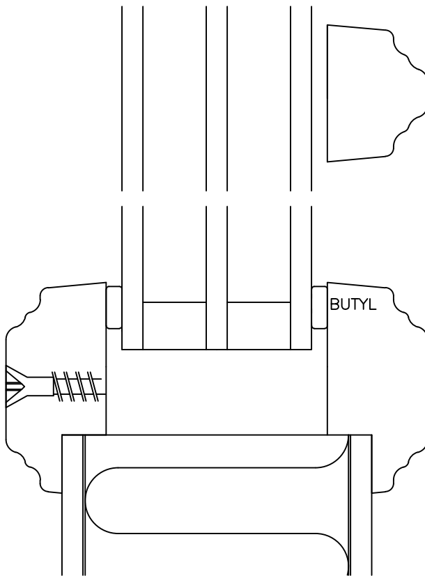
SNITT A-A
